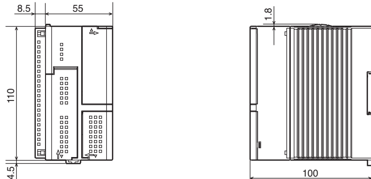
CPU Module
